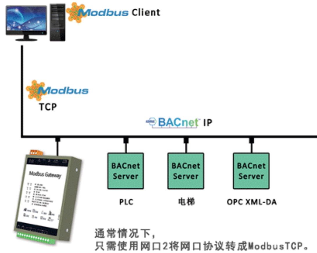
场景1: 集成网口协议 (以BACnetIP为例) 到ModbusTCP
