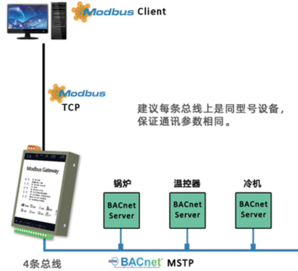
场景2: 集成串口协议 (以BACnetMSTP为例) 到ModbusTCP
